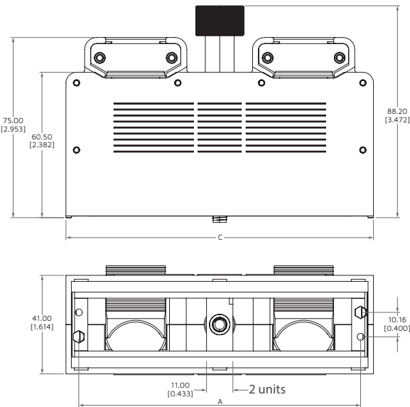
LEMVS Receptacle
