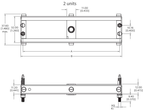
LEMVS Receptacle
